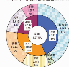
エネルギー消費の構成(全国2010FY)
