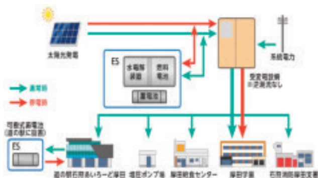
※報告文参照 石狩市厚田マイクログリッドシステムの概要 (緑→：通常時、赤→：停電時)
