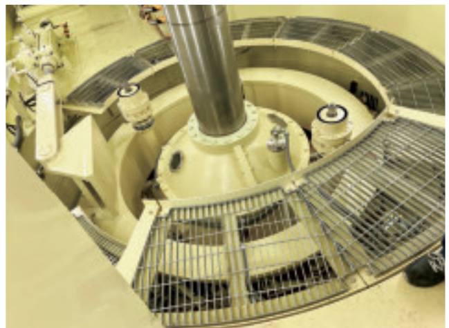
清水沢ダム 発電機の駆動部分
