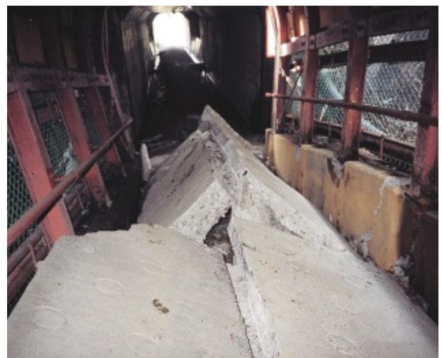
川口駅横断地下通路の損壊
