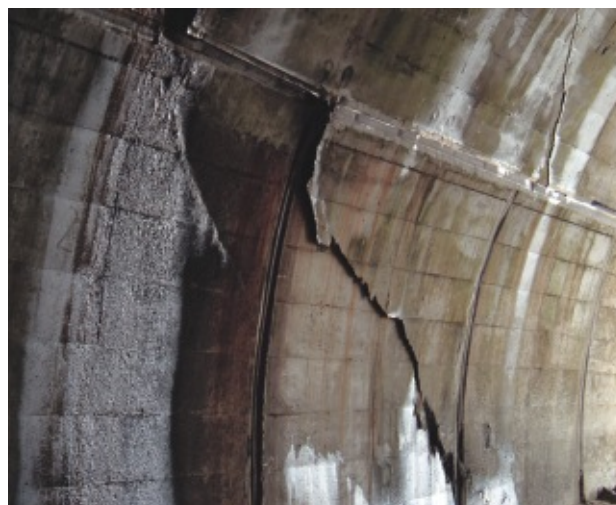
県道荒谷トンネル 斜め亀裂
