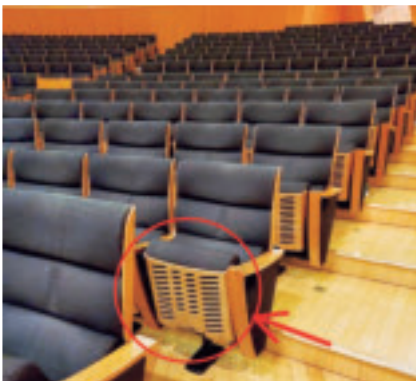
客席裏側の穴 有害エコーを吸音する
