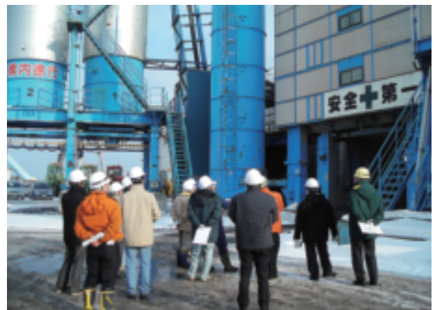
アスファルトプラント(120 t/h)
